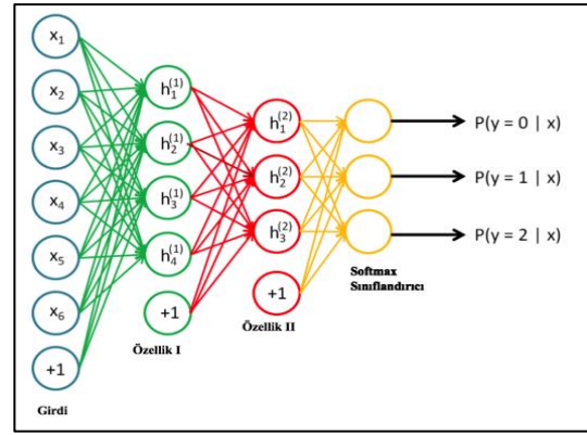
Şekil 5. Genel bir DAE mimarisi [76].
