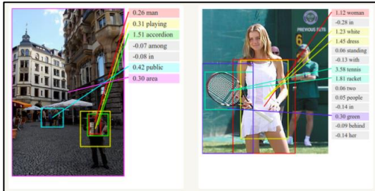
Şekil 4. Görüntü tanımlayıcıları oluşturmak için derin görsel-anlamsal hizalama [43].
